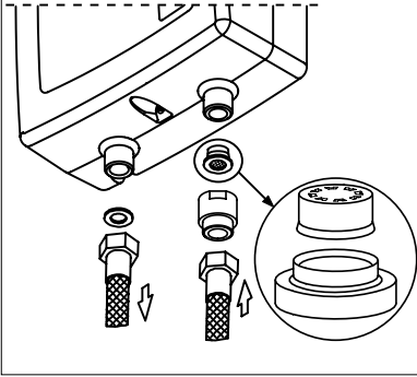
Montage mit Stutzen nach unten gerichtet
