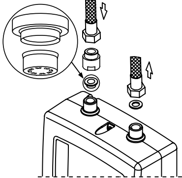
Montage mit Stutzen nach oben gerichtet
